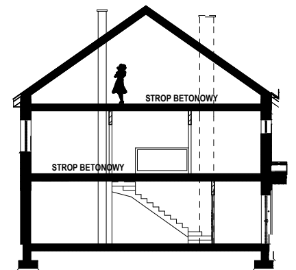
PRZEKRÓJ
