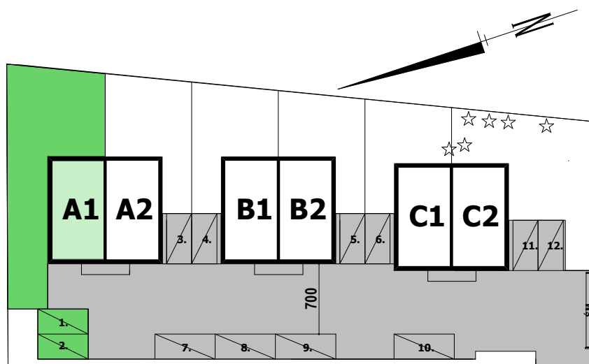
ZAGOSPODAROWANIE TERENU
