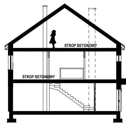
PRZEKRÓJ
