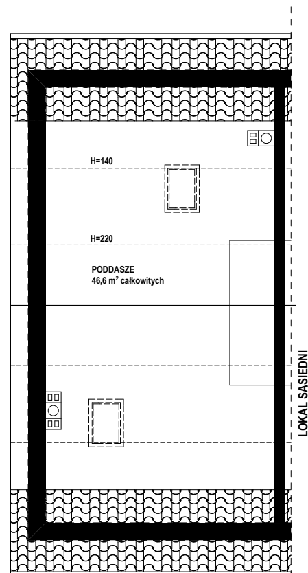
PODDASZE
